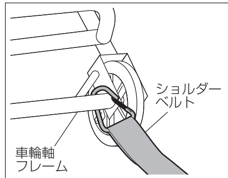
ショルダーベルト取付け （車輪軸フレーム部分）
