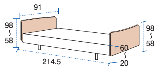
ベッド寸法図 (cm)
